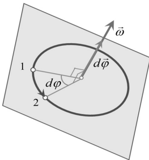
Նկ.2-6 Անկյունային տեղափոխության և անկյունային արագության վեկտորները:
