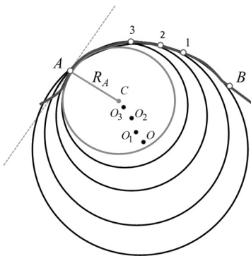
Նկ.1-10 Կորության կենտրոն և կորության շառավիղ:
