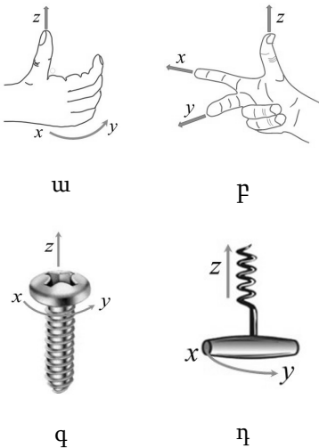
Նկ.1-2 Աջ համակարգ:
