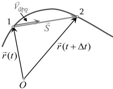
Նկ. 2-1 Տեղափոխության և միջին արագության վեկտորները:
